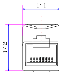
8P8C
